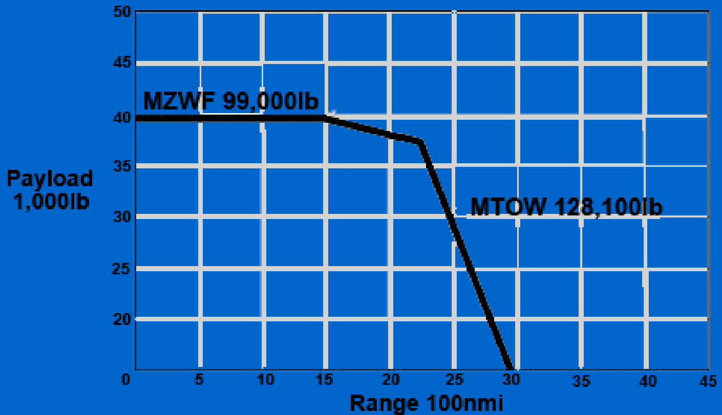
Boeing 737-200 Cargo
